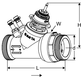
DN 40-50 HP – Temperatur -10 – +90°C, \Delta pV max. 600 kPa Außengewinde gemäß ISO 228
