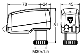
TA-Slider 500 I/O Sygnał sterujący: 0(2)-10 VDC
