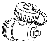
Zawór do napełniania, opróżniania, płukania i odpowietrzania przyłączy 1/2"
