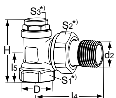
Vinkel inkl radiatorforskruing
