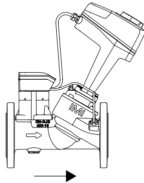
DN 65-150
