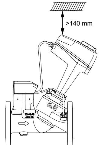
DN 65-150
