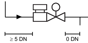
DN 65-150
