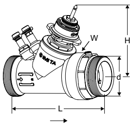
DN 40-50 HP – Temperatuur -10 – +90°C, \Delta pV max. 600 kPa Buitendraad volgens ISO 228
