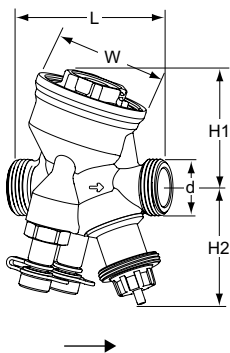
DN 10-32 HP – Temperatuur -20 – +120°C, \Delta pV max. 600 kPa Buitendraad volgens ISO 228
