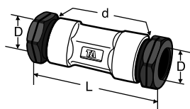
Suora liitin Du x Du
