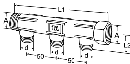
3-haarainen jakotukki Varustettuna vapaasti kiertyvällä mutterilla
