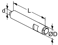
Luftpunktsforlengelse Benyttes når ventilen skal isoleres. Rustfritt stål/EPDM/Messing.
