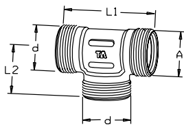
TA 352 Trójniki GZ
