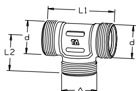
TA 352 Trójniki GZ
