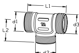
TA 352 Trójniki
