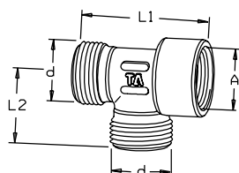
TA 362 Trójniki GW
