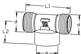
TA 362 Trójniki GW
