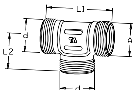
TA 352 Trójniki
