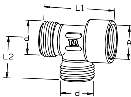
TA 362 Trójniki GW
