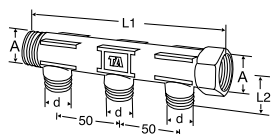
TA 56 043, Rozdzielacz 3-obwodowy Z nakrętką
