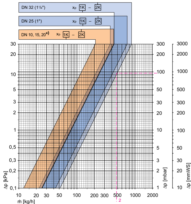
Diagram DN 10 (3/8") axiální, DN 10 (3/8") a DN 15 (1/2") úhlový, DN 20 (3/4") plošně těsnící, DN 25 (1") a DN 32 (1 1/4"), radiátorový ventil s termostatickou hlavicí
