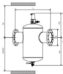
Separátor nečistôt
