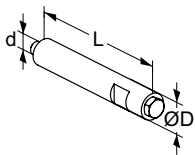
Predĺženie odvzdušnenia Vhodné pri použití izolácie. Nehrdzavejúca ocel/EPDM/Mosadz.
