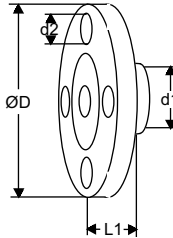
Pripojenie s prírubou Prírubby podľa EN-1092-2:1997, typ 16.
