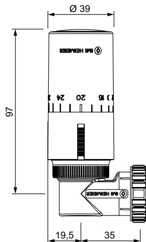
Nurkühendus koos termostaatpeaga D
