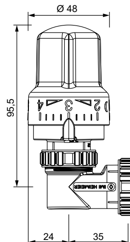
Nurkühendus koos termostaatpeaga S
