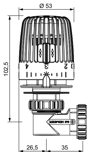
Nurkühendus koos termostaatpeaga DX
