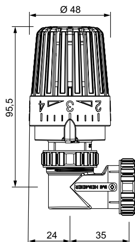
Nurkühendus koos termostaatpeaga D
