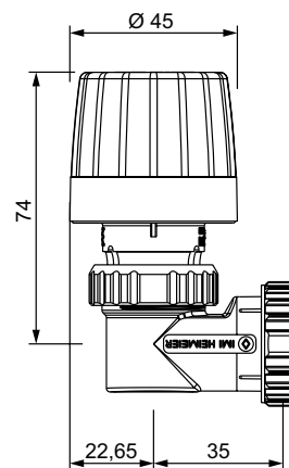
Nurkühendus koos EMOfec
