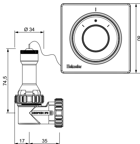
Nurkühendus koos termostaatpeaga F
