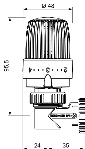
Nurkühendus koos termostaatpeaga S
