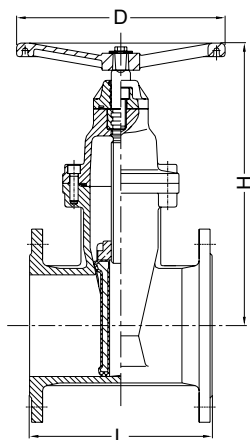
Фланцевое С рукояткой
