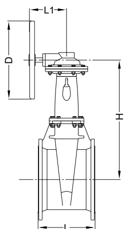
Фланцевое С редуктором
