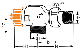
Axial mit Außengewinde G 3/4
