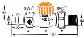
Durchgang mit Viega Pressanschluss 15 mm
