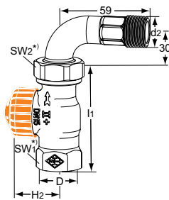
Durchgang mit Bogenverschraubung
