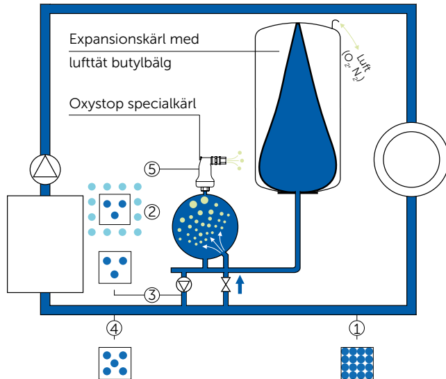
Förbättrad Pneumatex-lösning med lufttät teknik. Ingen avgasning i expansionskärl elimineras risken för syrgasdiffusion
