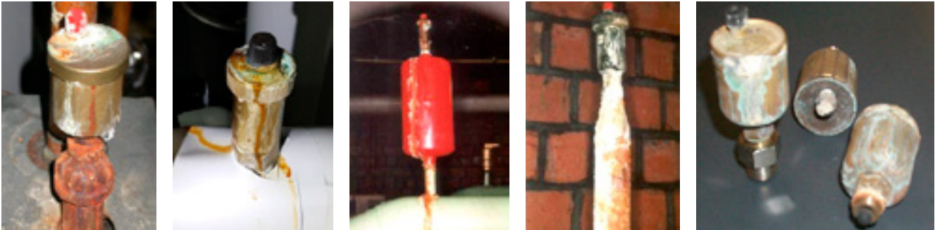
Exempel på luftavskiljare som börjar läcka pga felaktig konstruktion
