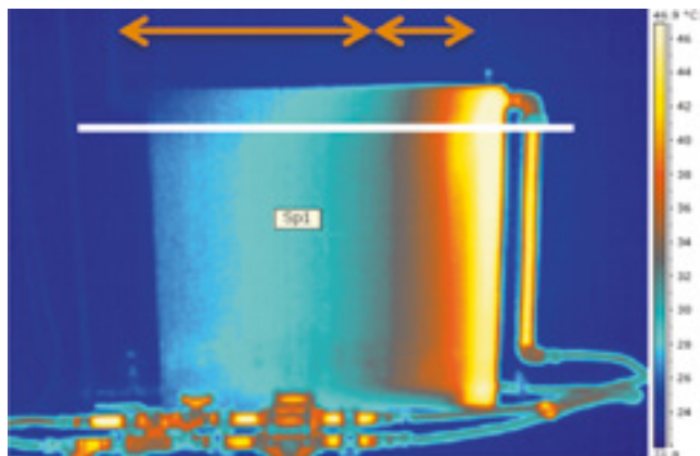
Luftens påverkan på radiatorns avgivna effekt (*)
