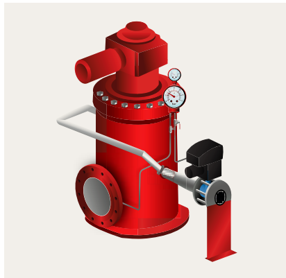
Automatiskt filter
