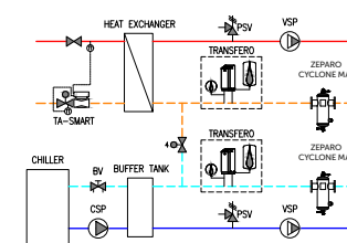
Système change-over avec comptage d'énergie par zone
