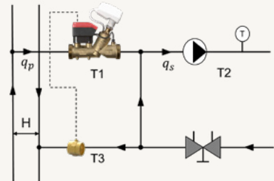
Régulation circuit secondaire / tertiaire
