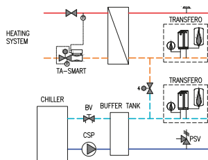
Système change-over
