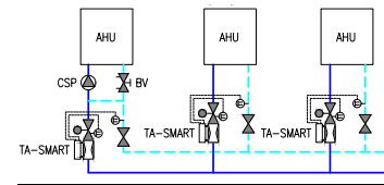
Système de refroidissement – débit variable
