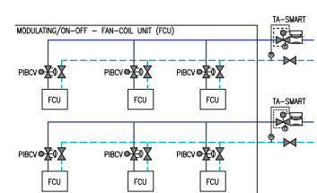
Système de refroidissement – vanne de zone
