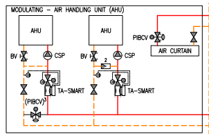
Système de chauffage – débit variable
