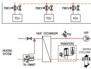
Système de chauffage – avec comptage d'énergie par zone
