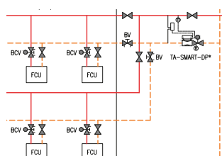
Système de chauffage - Contrôle de la pression
