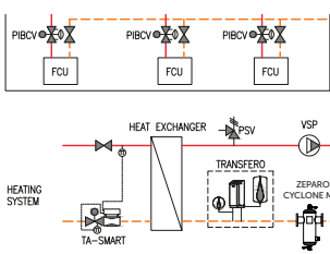
Impianto di riscaldamento – Valvola di zona
