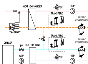
Impianto a 4 tubi – Valvola di zona
