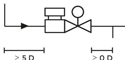
TA-Smart DN65-125
