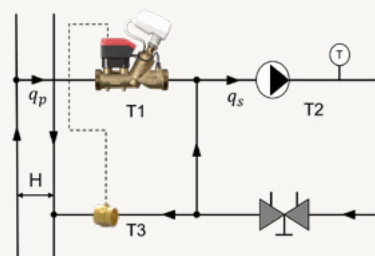
Controllo circuito secondario / terziario
