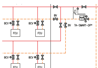
Sistema di riscaldamento – Controllo della pressione
