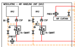
Impianto di riscaldamento – Portata variabile
