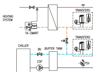
Impianto a 4 tubi – Portata variabile
