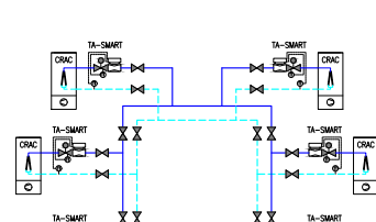
Unità CRAC – Portata variabile
